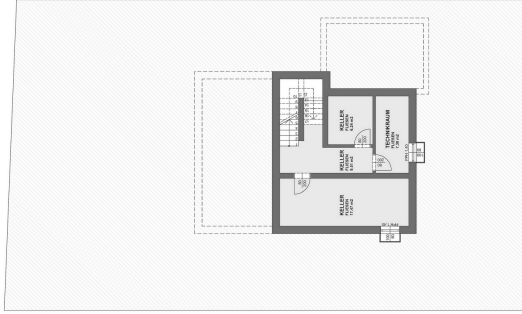
HAUS TYP 2 - KELLERGEHOSS OPTIONAL
